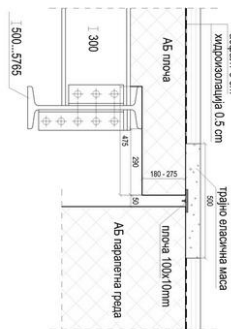
ПРЕСЕК В ДЕТАЉ АСФАЛТНЕ ДИЛАТАЦИЈЕ КОД СТУБА S2 Р 1:10
