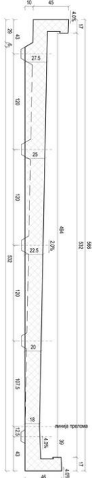
ПРЕСЕК 3-3 Р 120
