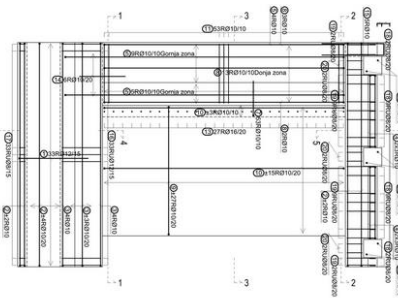
ПЛАН АРМАТУРЕ НОВИХ БЕТОНСКИХ ЕЛЕМЕНАТА НА СТУБ S2 P 1:50
