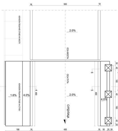
СТУБ S2 - ПОГЛЕД ОДОЗГО P 1:50
