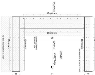
ПЛАН АНКЕРА ЗА БЕЗУ НОВИХ БЕТОНСКИХ ЕЛЕМЕНАТА НА СТУБ S2 P 1:50
