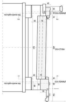
ИЗГЛЕД СТУБА S2 P 1:50
