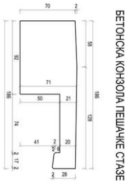
ПРЕСЕК 4-4 P 1:20
