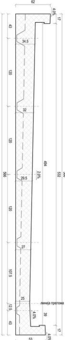
ПРЕСЕК 5-5 Р 120
