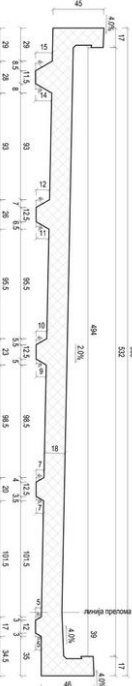
ПРЕСЕК 1-1 Р 120
