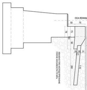
ПРЕСЕК 2-2 P 1:50
