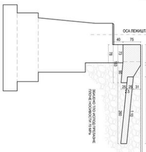
ПРЕСЕК 1-1 P 1:50
