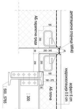
ПРЕСЕК А ДЕТАЉ ДИЛАТАЦИОНЕ СПОЈНИЦЕ МР-40 КОД СТУБА S1 Р 1:10
