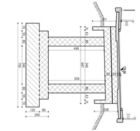
СТУБ С5 - ПРЕСЕК 7-7 P 1:100
