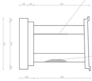
ПРЕСЕК 4-4
