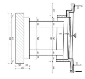
СТУБ С5 - ПРЕСЕК 8-8 P 1:100
