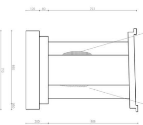
ПРЕСЕК 6-6
