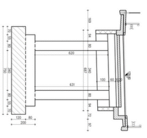
СТУБ С1 - ПРЕСЕК 2-2 P 1:100
