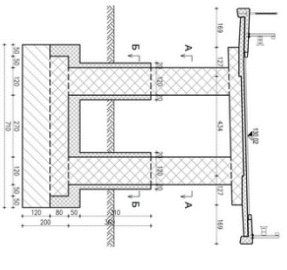
СТУБ С2 - ПРЕСЕК 4-4 P 1:100
