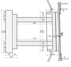
СТУБ С1 - ПРЕСЕК 3-3 P 1:100
