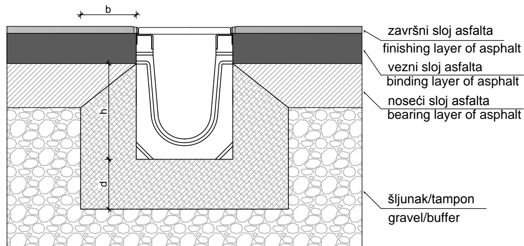
DETALJ UGRADNJE KANALETE U ASFALTNOJ POVRŠINI DETAIL DRAWING OF DRAIN CHANNEL IN ASPHALT SURFACE
