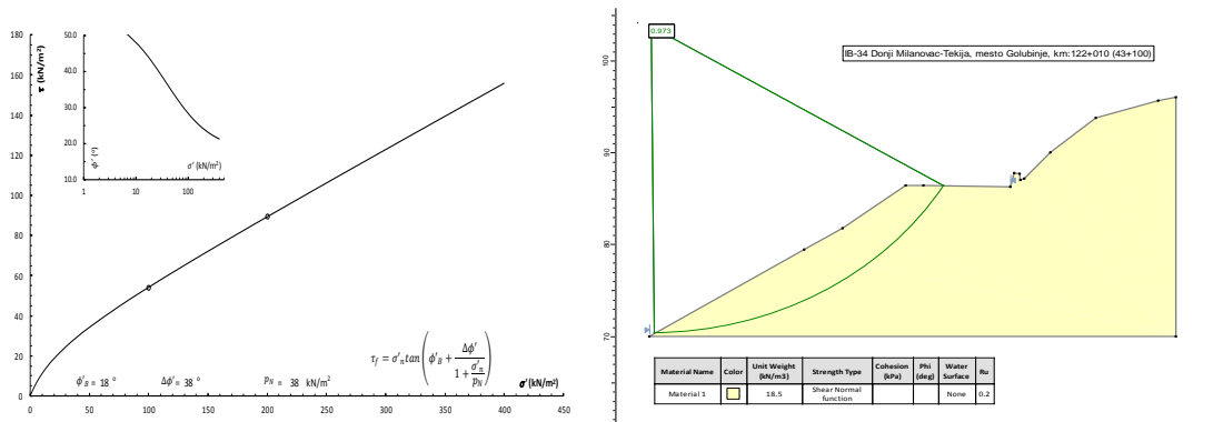
Слика 2. Анализа стабилности косине дуж геотехничког пресека терена - 0+090
