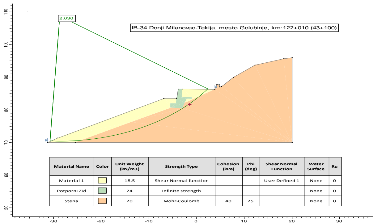
Слика 3. Анализа стабилности косине дуж геотехничког пресека терена - 0+090 после санације
