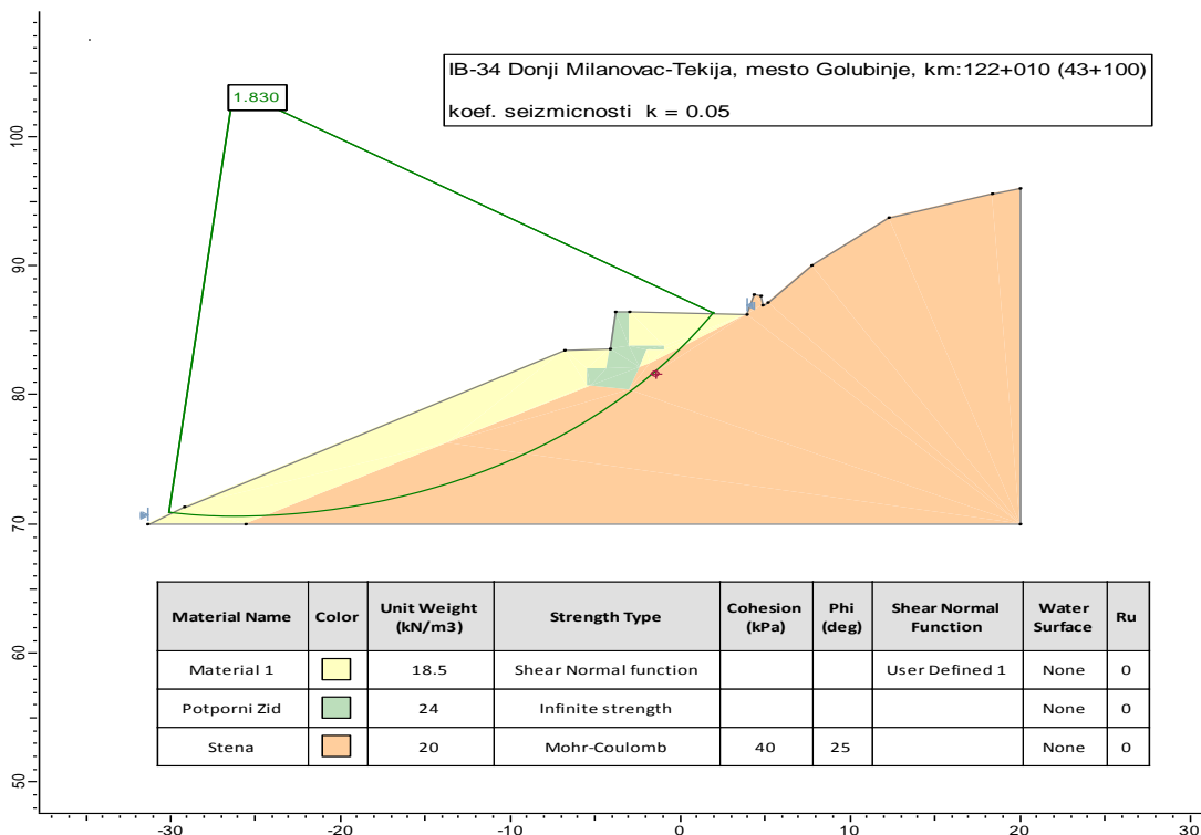
Слика 5. Анализа стабилности косине дуж геотехничког пресека терена - 0+090 после санације, утицај земљотреса
