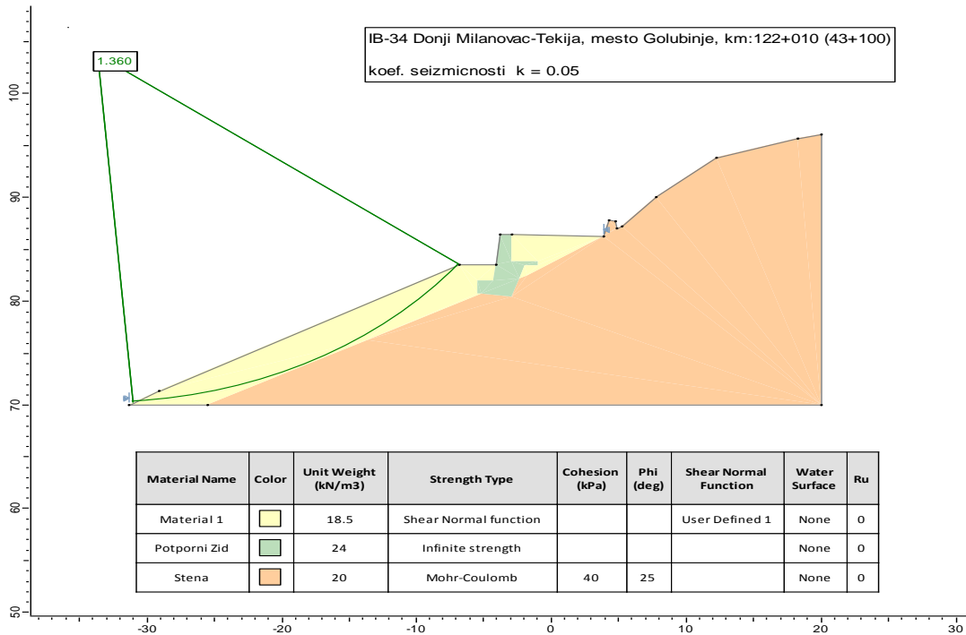
Слика 6. Анализа стабилности косине испред зида, дуж геотехничког пресека терена - 0+090 после санације, утицај земљотреса
