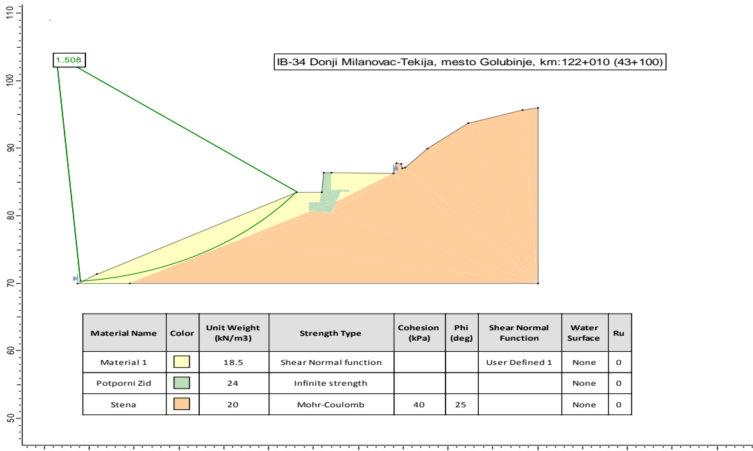
Слика 4. Анализа стабилности косине испред зида, дуж геотехничког пресека терена - 0+090 после санације
