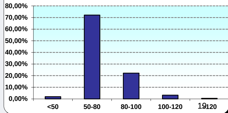
Дистрибуција брзина
