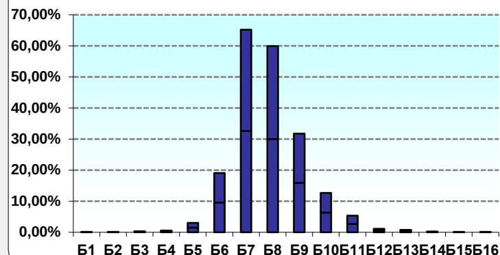
Дистрибуција брзина
